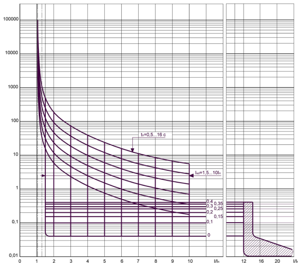
Рисунок 2 - Время-токовая характеристика выключателей
