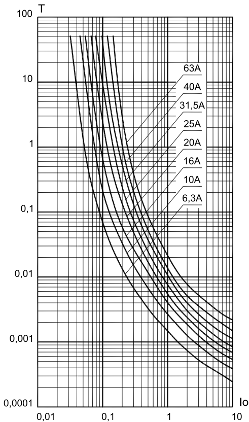
Рисунок В.5 – Преддуговые время-токовые характеристики при напряжении 220 В постоянного тока
