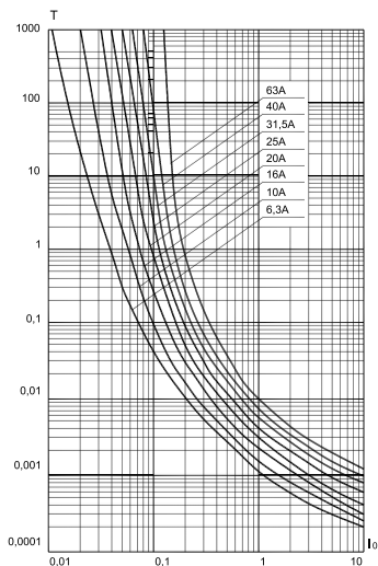
Рисунок В.2 – Предугуговые время-токовые характеристики при напряжениях 380 и 500 В переменного тока
