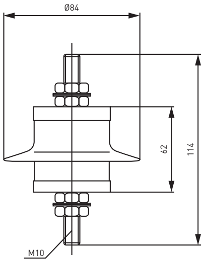
Рис. 2 - ОПН-П 0,66
