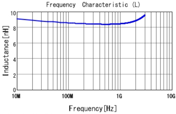
■ LQW15AN8N7H00 L
