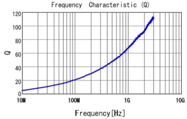
■ LQW15AN8N7H00 Q
