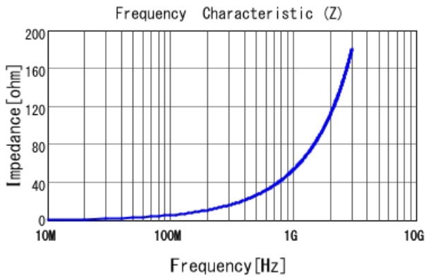
■ LQW15AN8N7H00 |Z|
