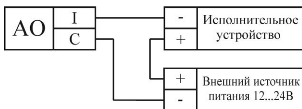
Рисунок 6 Подключение к модулю исполнительных механизмов с сигналом по току.
