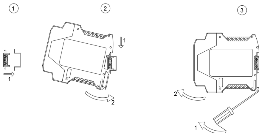
Рисунок 8 – Монтаж модуля на DIN-рейку и снятие модуля с неё.
