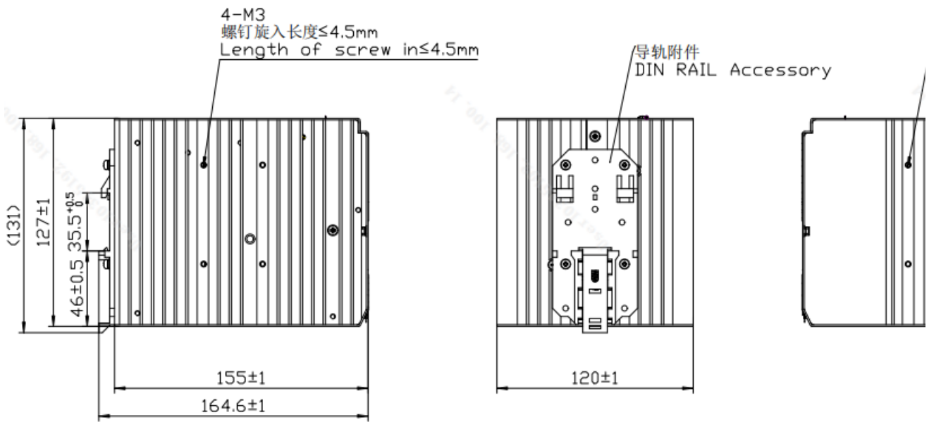
导轨电源SDP2-1AC24-960结构图
