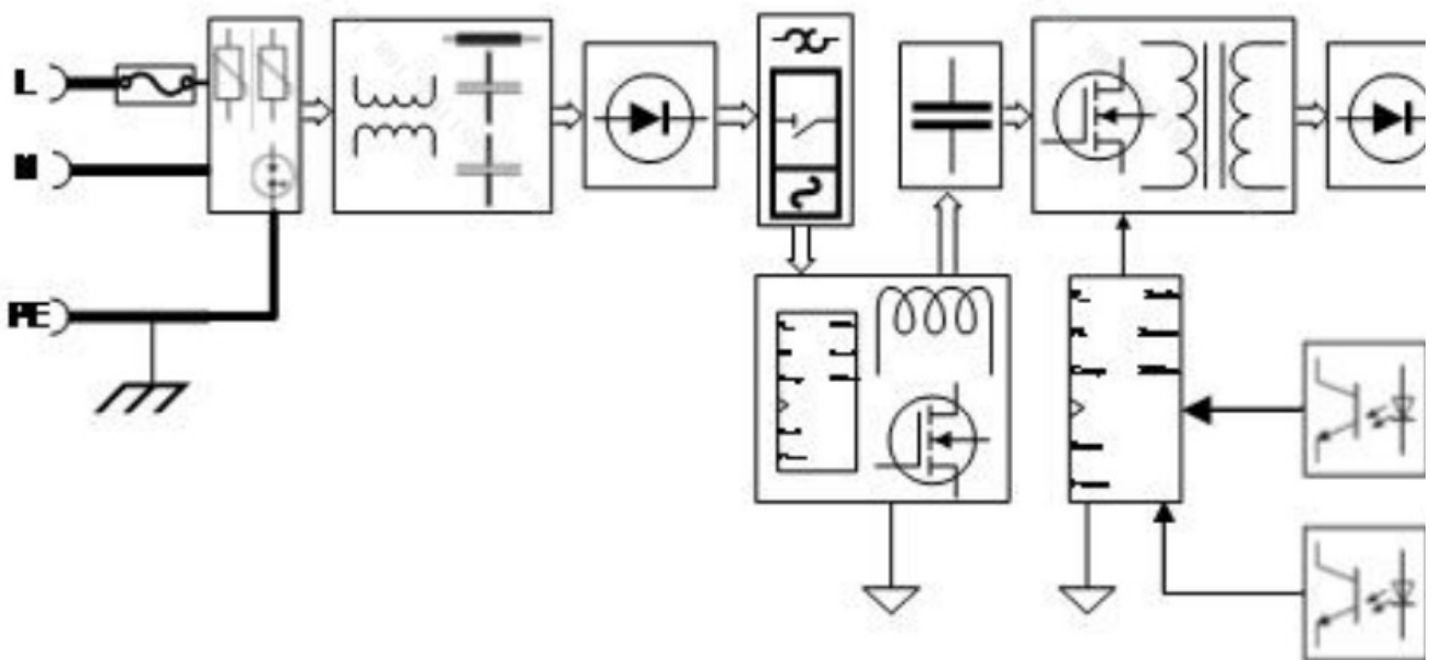
导轨电源SDP2-1AC24-960电气图
