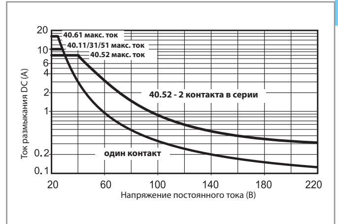
Н 40.2 - Макс. отключающая способность DC1 Типы 40.31/51/52/61 (страница 4) и 40.11 (страница <?>)
