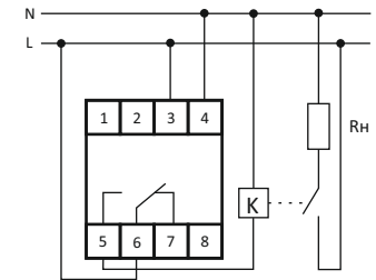
Rn - подключаемая нагрузка
