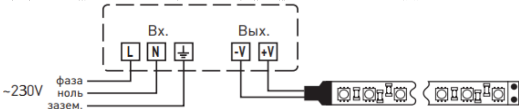
Рисунок 1 – Схема подключения
