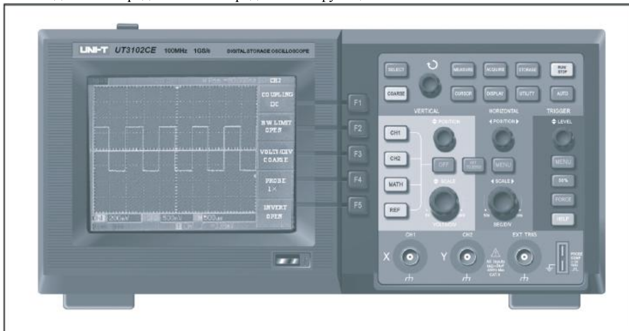
Рис.1-1 Передняя панель цифрового осциллографа серии UT2000E/3000E
