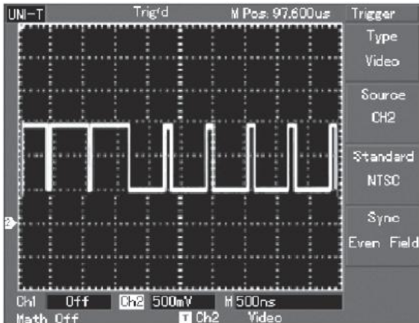
Рис. 2-15 Триггер видеосигнала: кадровая синхронизация
