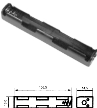
ВН-631 на 2 элемента "AA"
