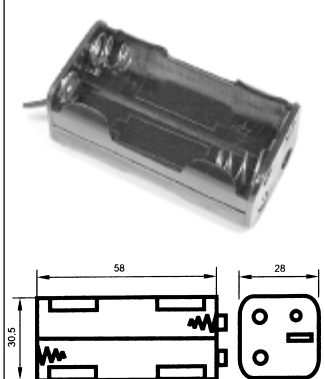
ВН-604 на 4 элемента "AA"
