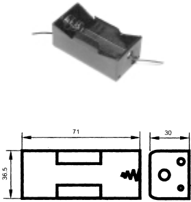
ВН-617 на 1 элемент "C"
