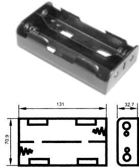
ВН-612 на 4 элемента "D"
