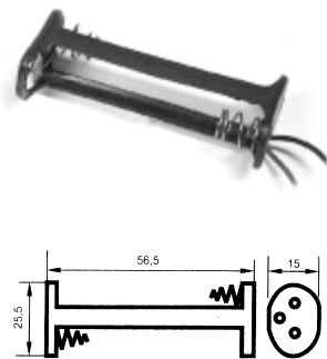
ВН-615 на 3 элемента "AA"
