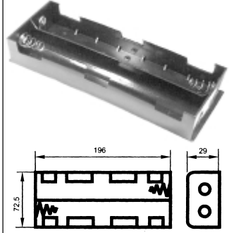
ВН-620 на 6 элементов "D"
