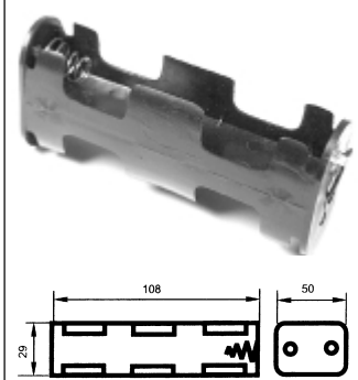
ВН-619 на 4 элемента "C"
