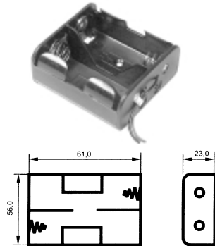
ВН-601 на 2 элемента "AA"
